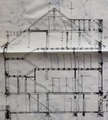
Querschnitt
