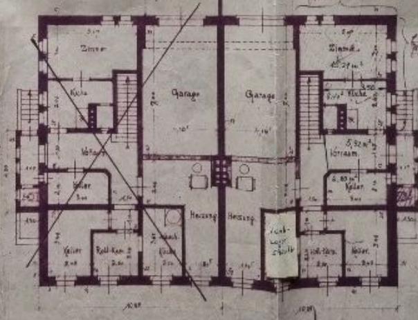
Kellergeschoss
